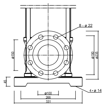
F(DIN) PN16 (DN100) /mm/
