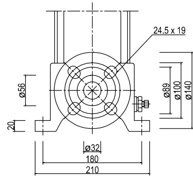
FGJ(DIN-ANSI-JIS) PN25(DN32) /mm/
