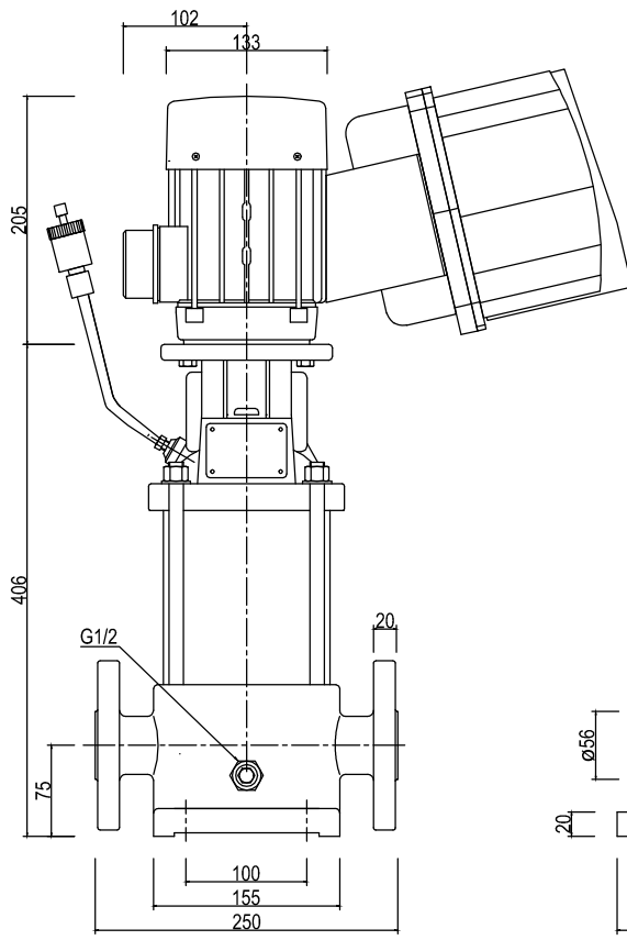
FGJ(DIN-ANSI-JIS) PN25(DN32) /mm/
