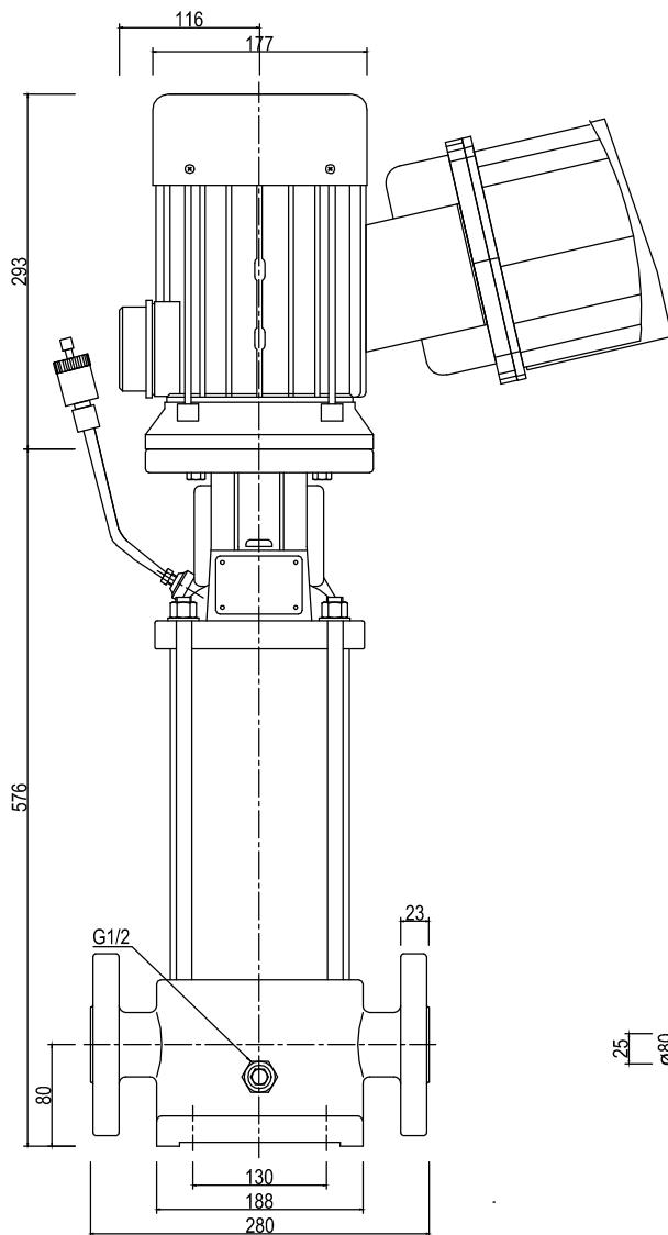
FGJ(DIN-ANSI-JIS) PN25(DN40) /mm/
