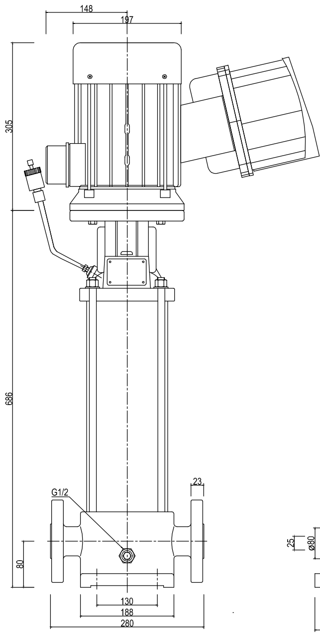
FGJ(DIN-ANSI-JIS) PN25(DN40) /mm/
